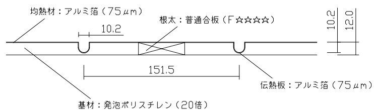
B-B'断面図
