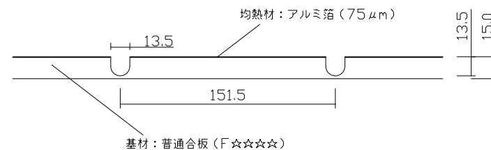
C-C'断面図
