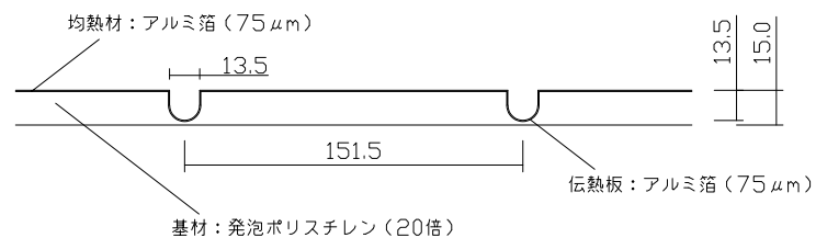
B-B'断面図
