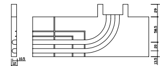
L 配管ガイドBL
