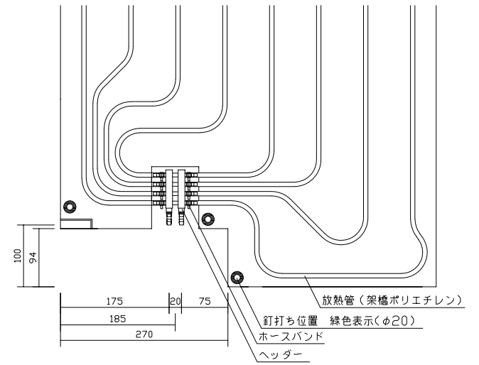
ヘッダー部拡大図
