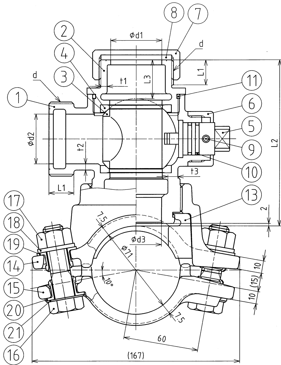
止水機構の寸法
