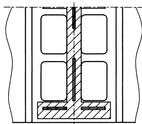
矢視 Z
