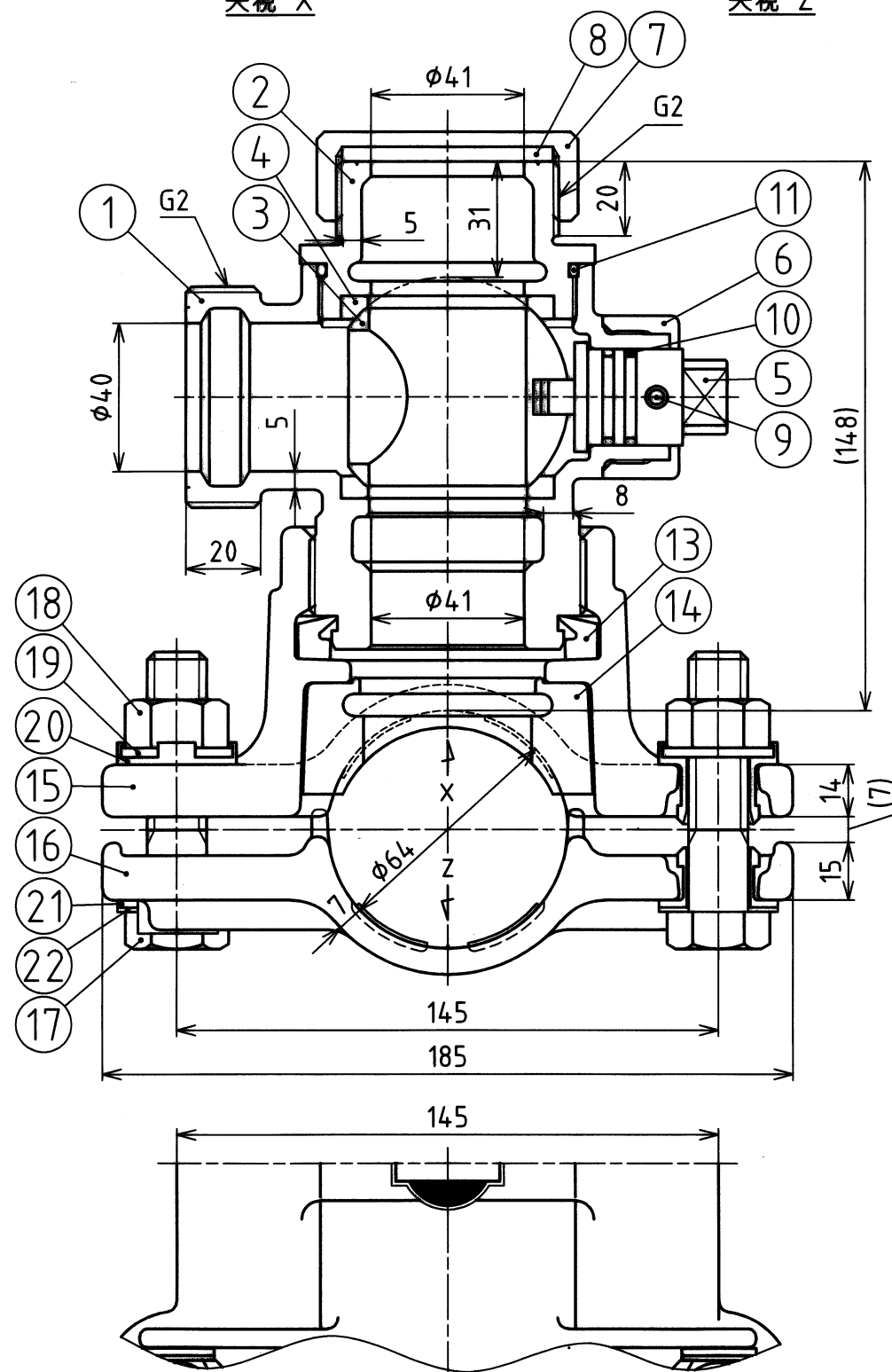
矢視 X
