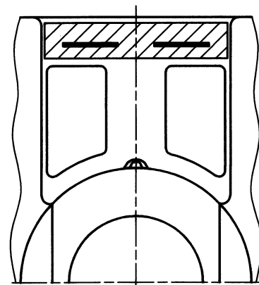
矢視 X
