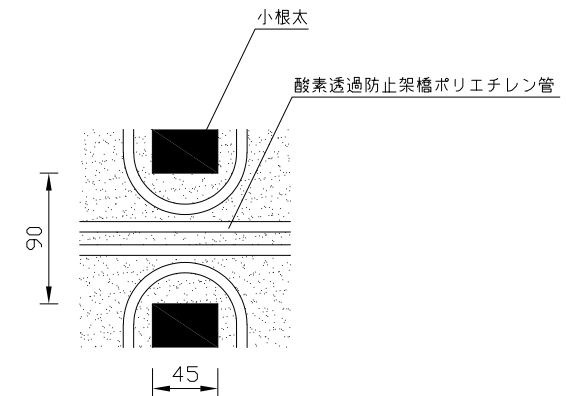
〈小根太一小根太間拡大図〉
