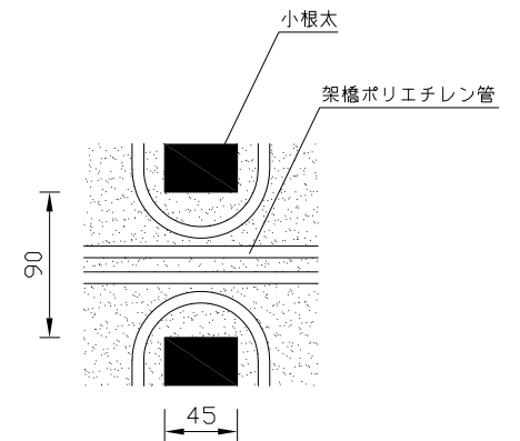
※2 小根太ー小根太間に「くぎ打ち禁止表示」
