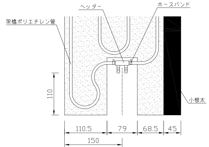
(小根太-小根太間拡大図)
