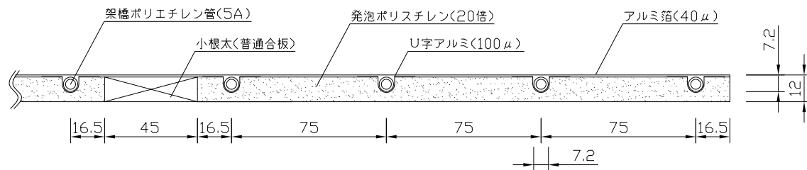
(A-A'断面図)
