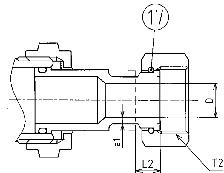
異径の場合
