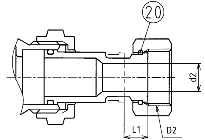
異径の場合
