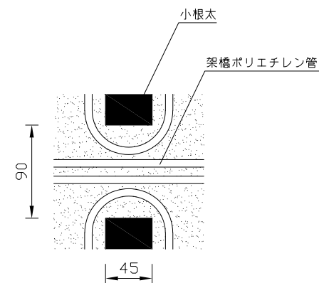
※2 小根太-小根太間に「くぎ打ち禁止表示」
