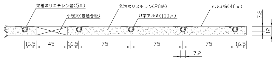
(A-A'断面図)
