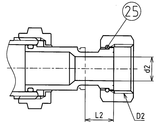
異径の場合
