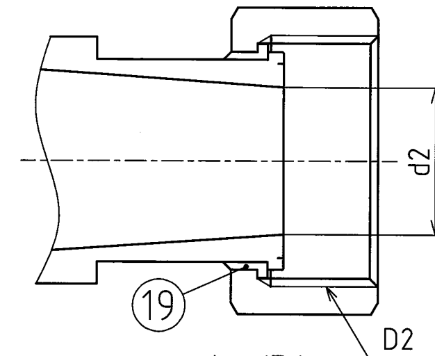
異径の場合
