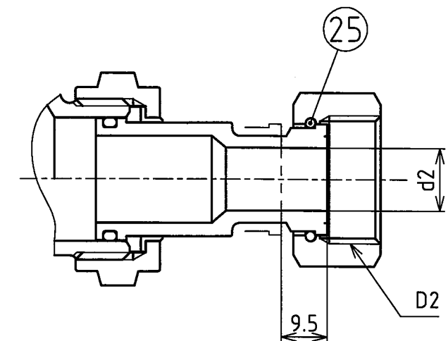
異径の場合
