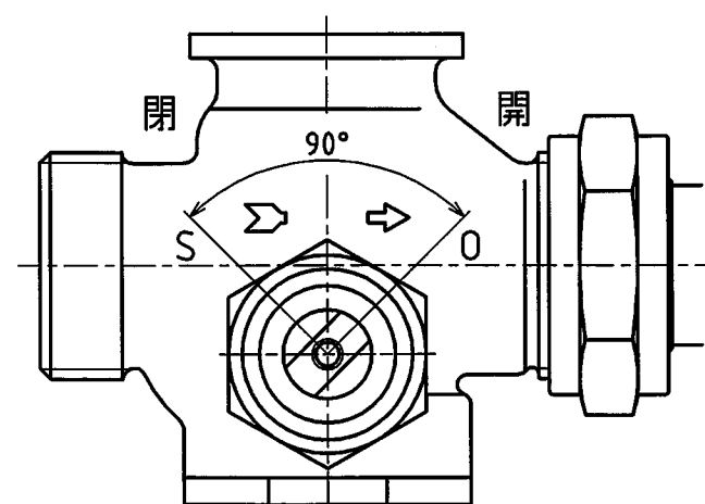
外観図(金属キャップを外した状態)
