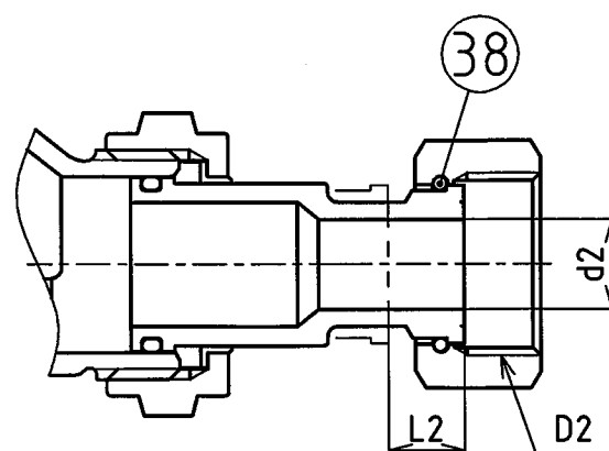
異径の場合
