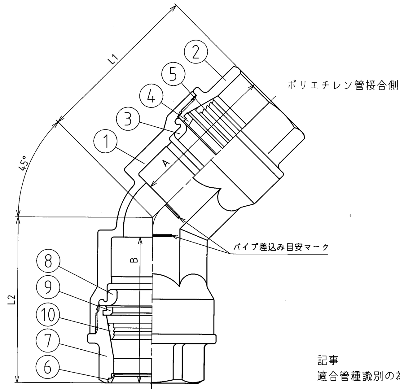
塩ビ管接合側
