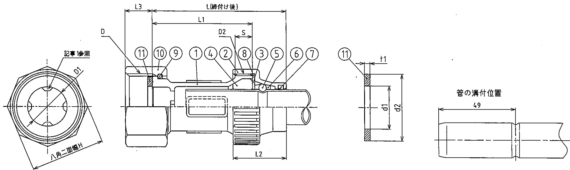
寸法表
