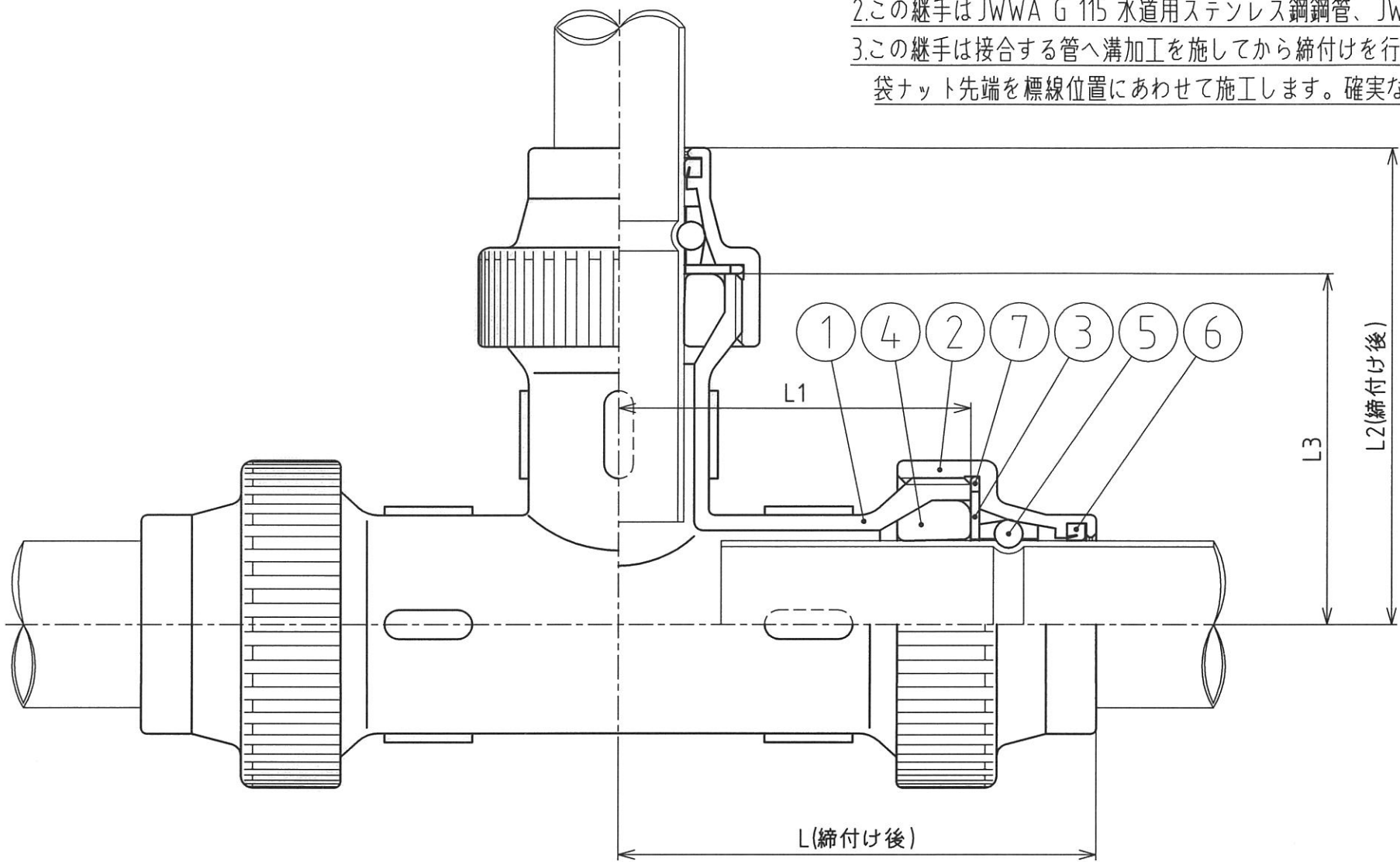
継手の寸法
