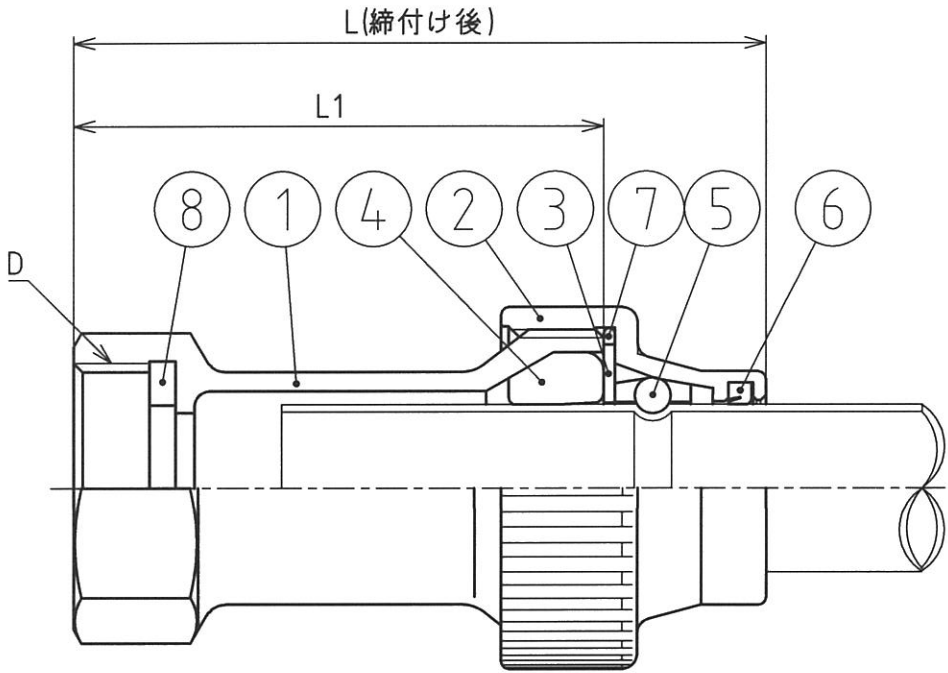
継手の寸法
