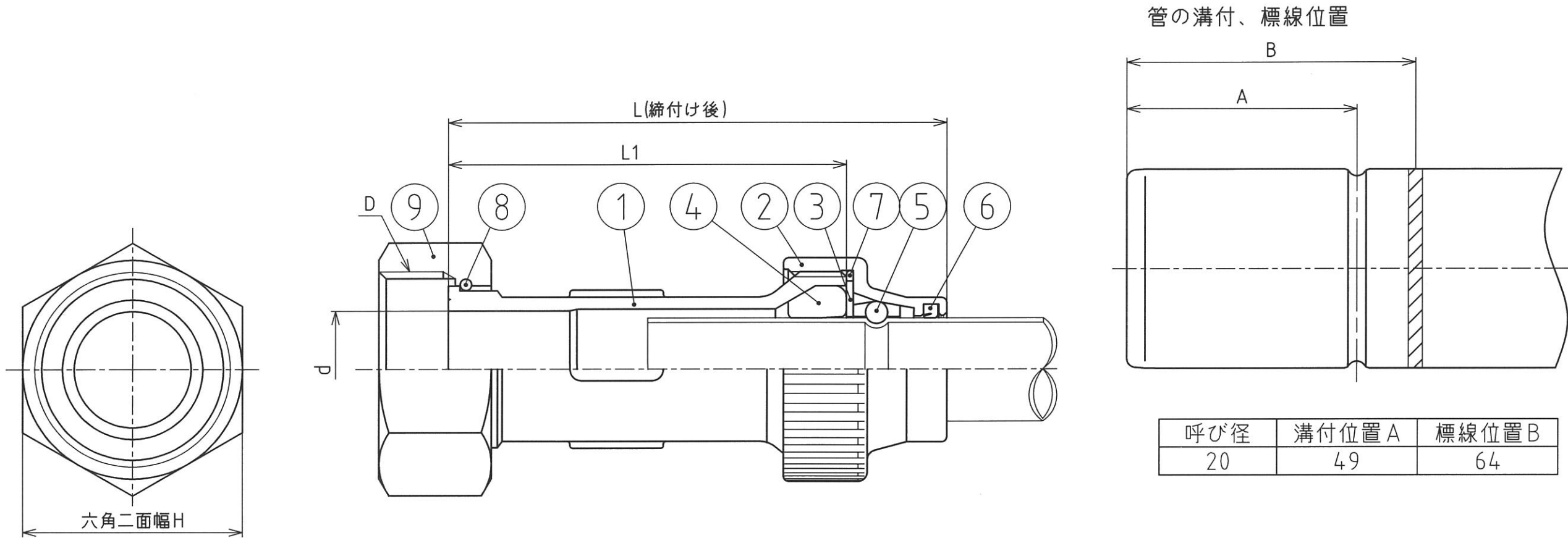
継手の寸法
