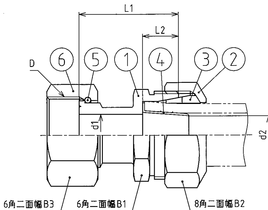
呼び径30のインコア形状
