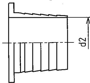
呼び径 40、50のインコア形状
