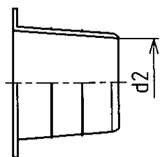
呼び径 25のインコア形状
