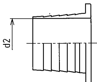
呼び径30~50のインコア形状
