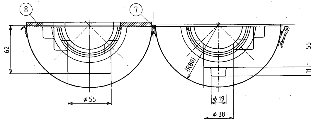
A-A断面
