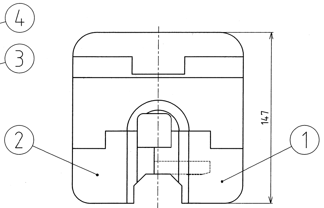
A矢視
