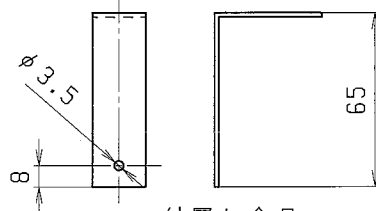
付属L金具 材質SECC 1.6t
