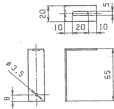
付属L金具 材質SECC 1.6t
