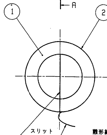
断面 A-A
