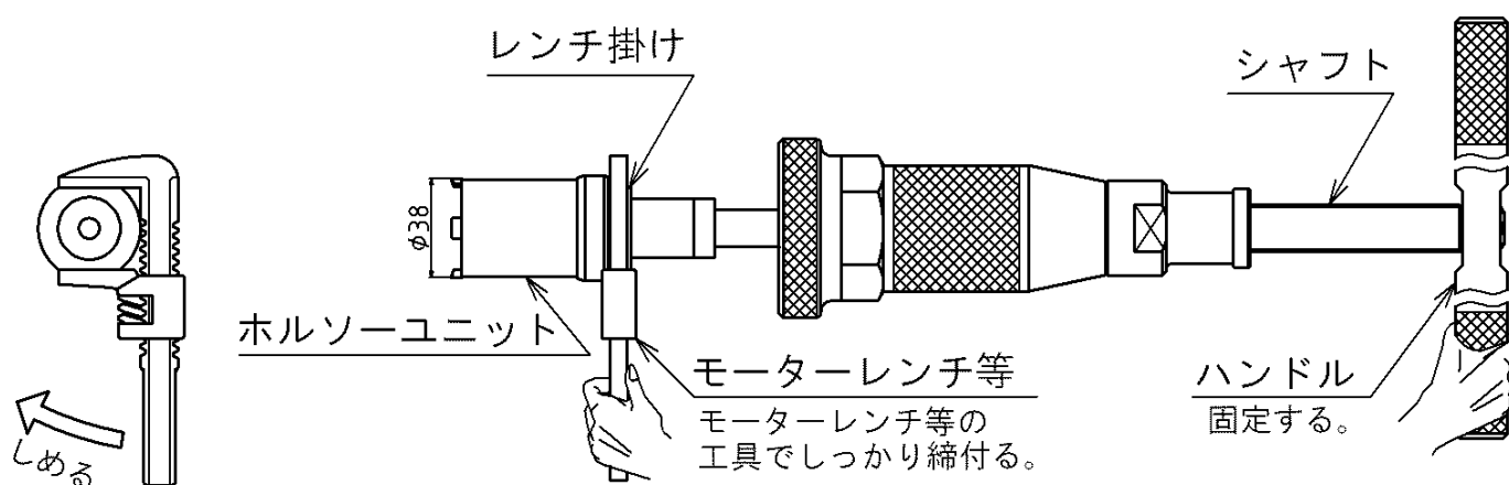
補足図 2 ホルソーユニット取り外し
