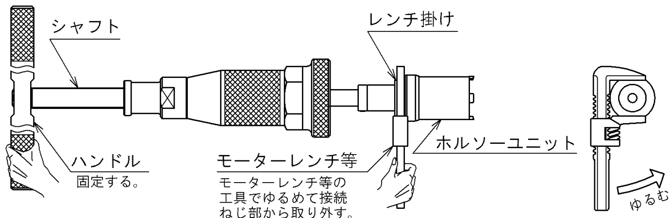
補足図 1 ホルソーユニット取り外し
