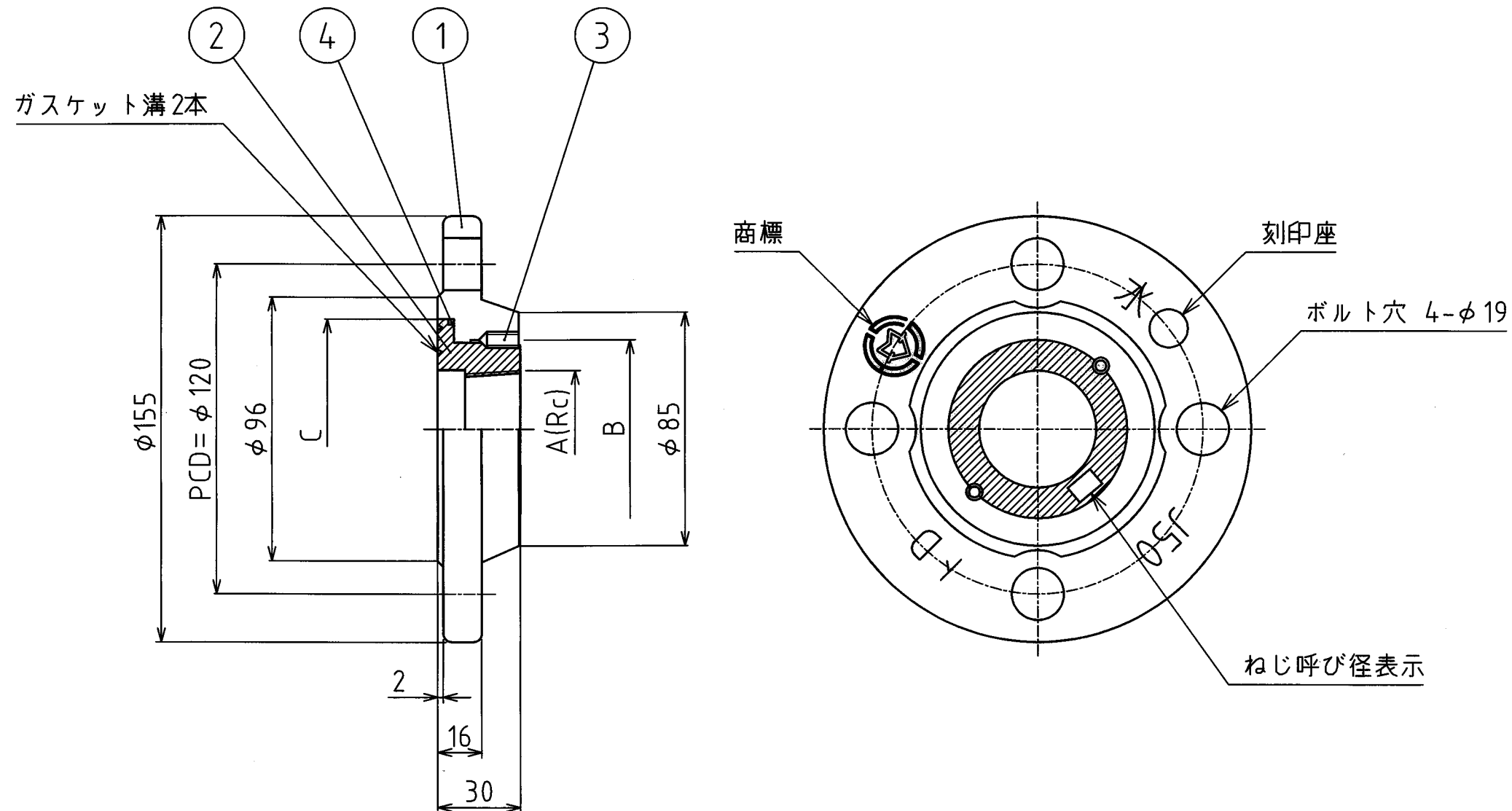
型式：SJFJ-50
